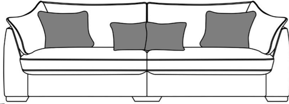
4 Seater Sofa 91cm (H) x 251cm (W) x 102cm (D) (Split-Frame Option Available) 3 Seater Sofa 91cm (H) x 221cm (W) x 102cm (D) (Split-Frame Option Available) 2 Seater Sofa 91cm (H) x 180cm (W) x 102cm (D) (Split-Frame Option Available)
